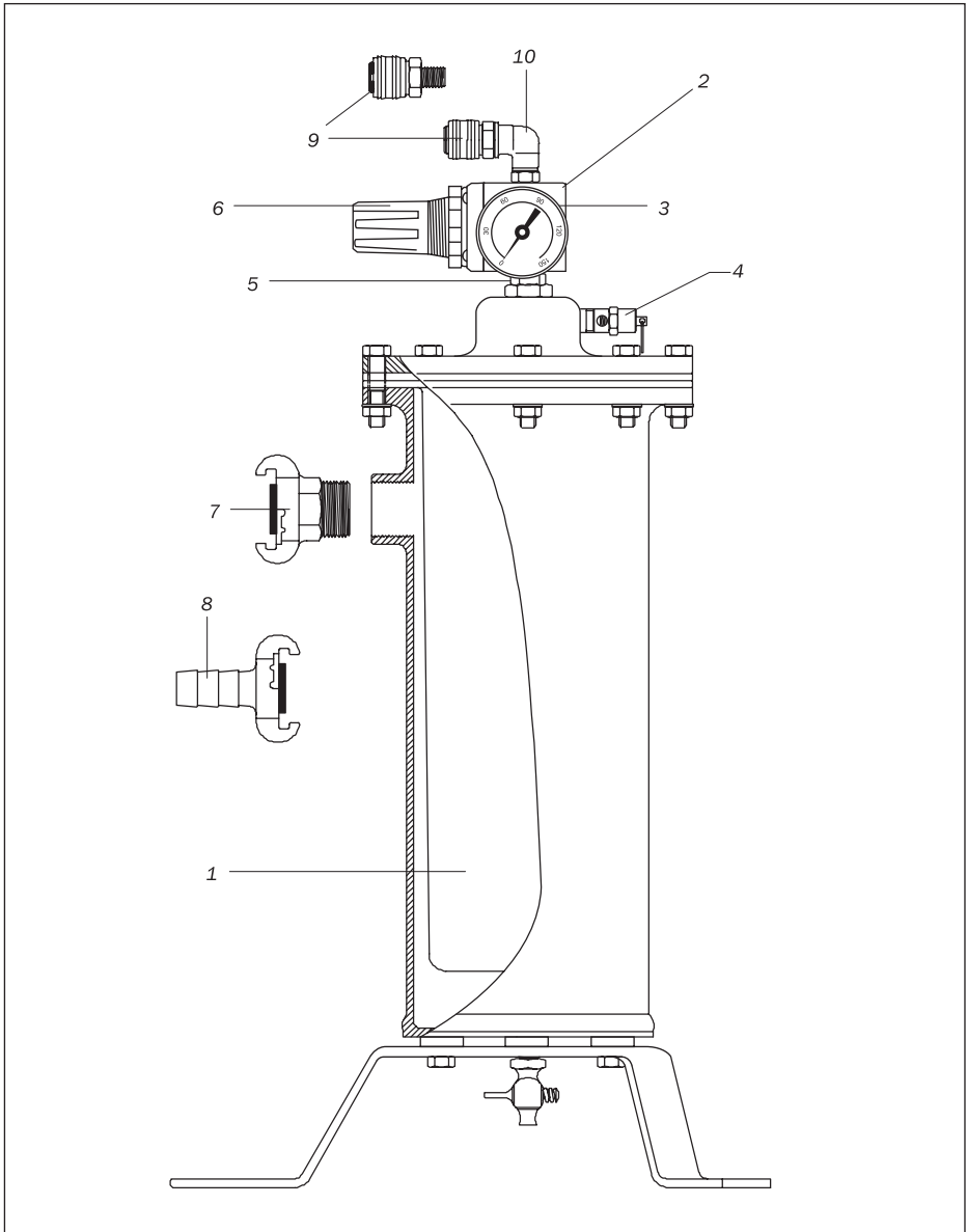
Abb. 2.1. Luftfilter BAF-1.
